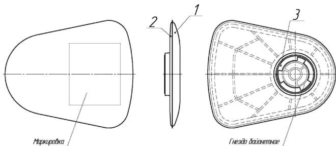
Рисунок 1 – Общий вид противоаэрозольного фильтра UNIX 203 P3 R D
